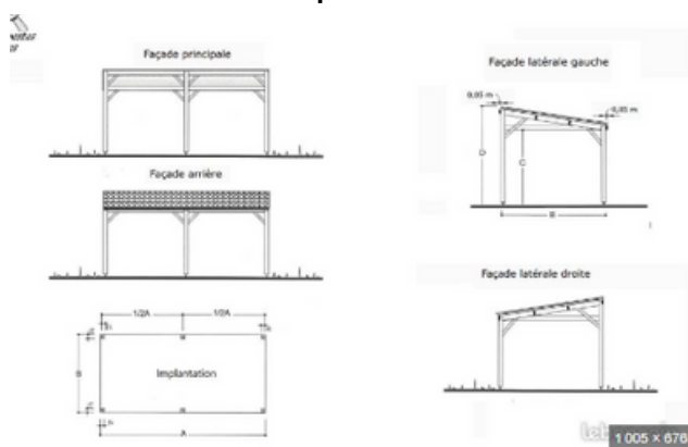
DPC 4 : élévation + toiture + coupes cotées
