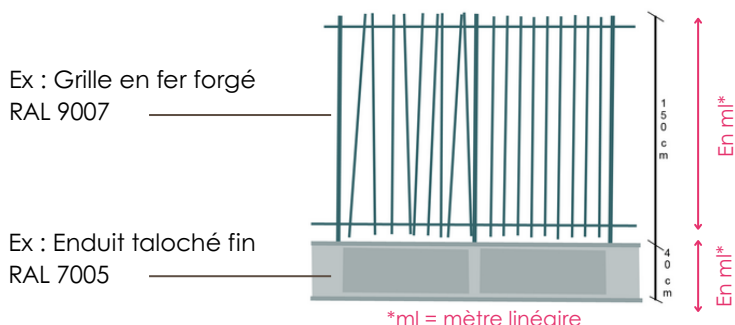
DPC 4 : élévation et coupes cotées
